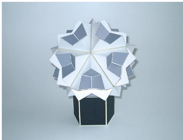
...umgestülpt zum Dual-TURINOS-Ikosaeder«
