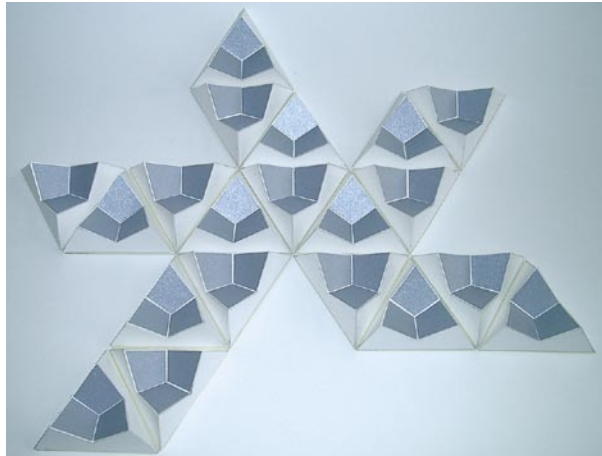
Die »Zentralabwicklung« des »Außen-Ikosaeders«...
