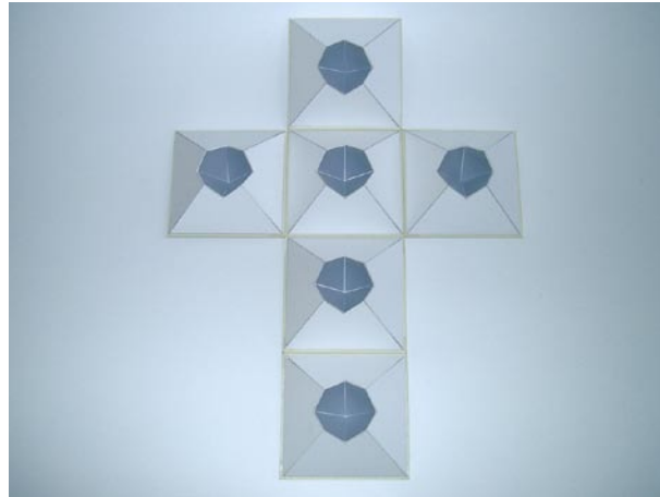
Die »Zentralabwicklung« des »Außen-Kubus«...
