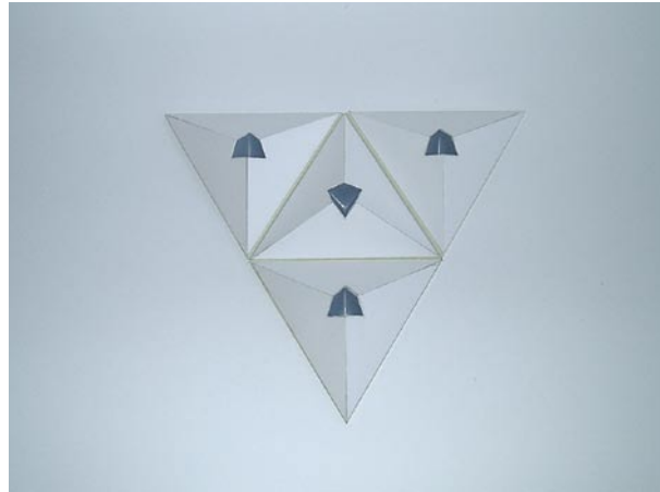
Die »Zentralabwicklung« des »Außen-Tetraeders«...
