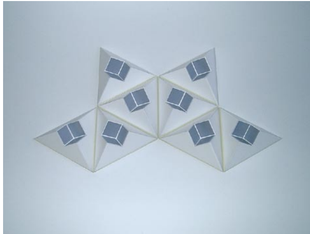
Die »Zentralabwicklung« des »Außen-Oktaeders«...
